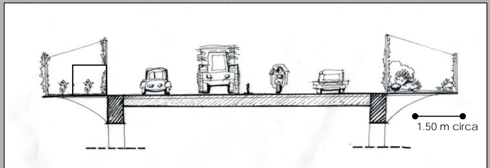
sezione trasversale
