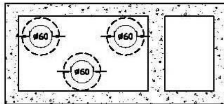
PARTICOLARE DI INSTALLAZIONE NUOVI CONDOTTI DI SCARICO FUMI
